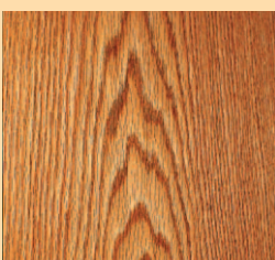
Roteiche
